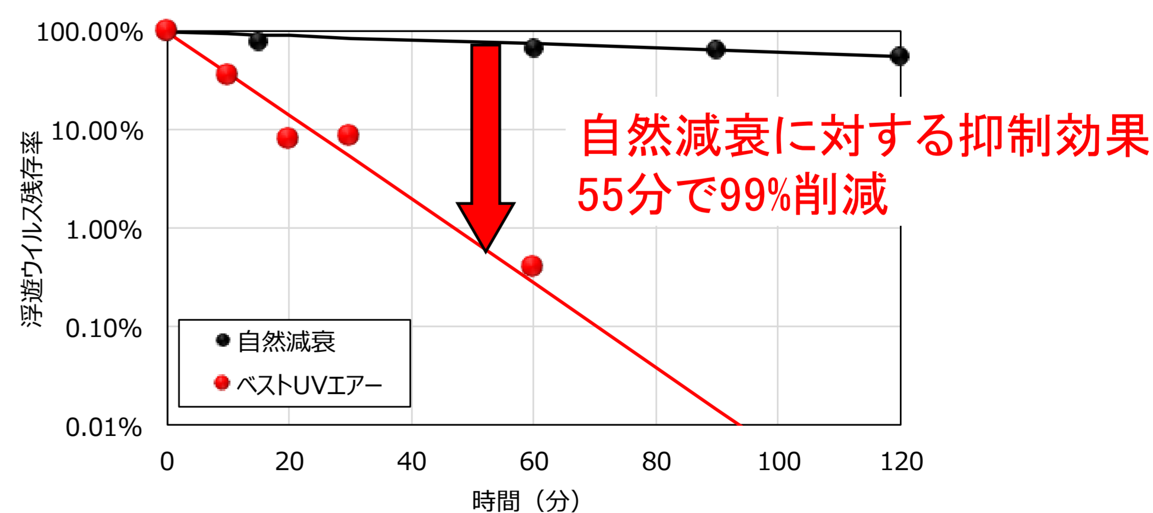
浮遊ウイルス削減効果(試験室での結果)
