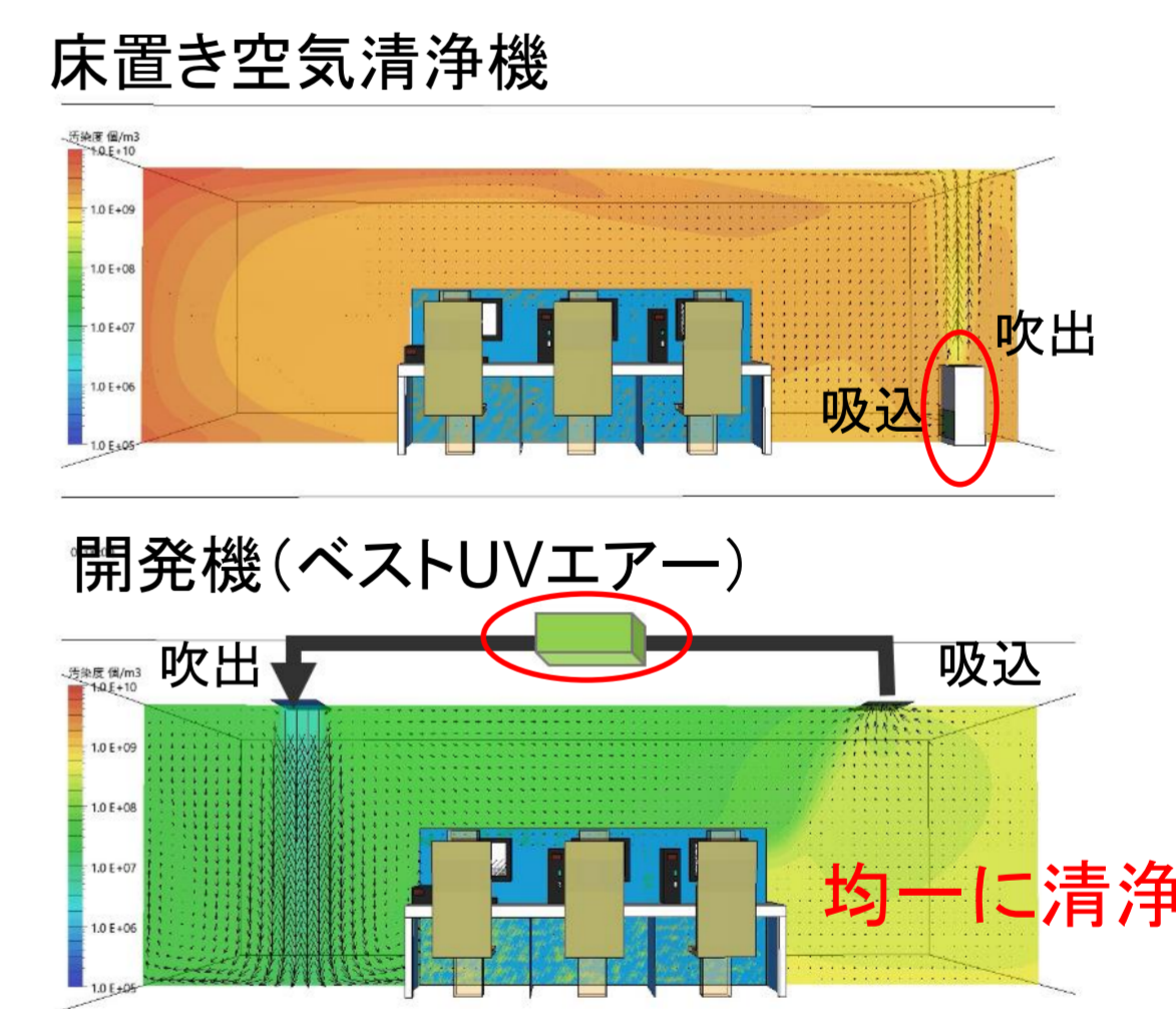
床置き空気清浄機と開発機の空気清浄状態の比較(シミュレーション)
